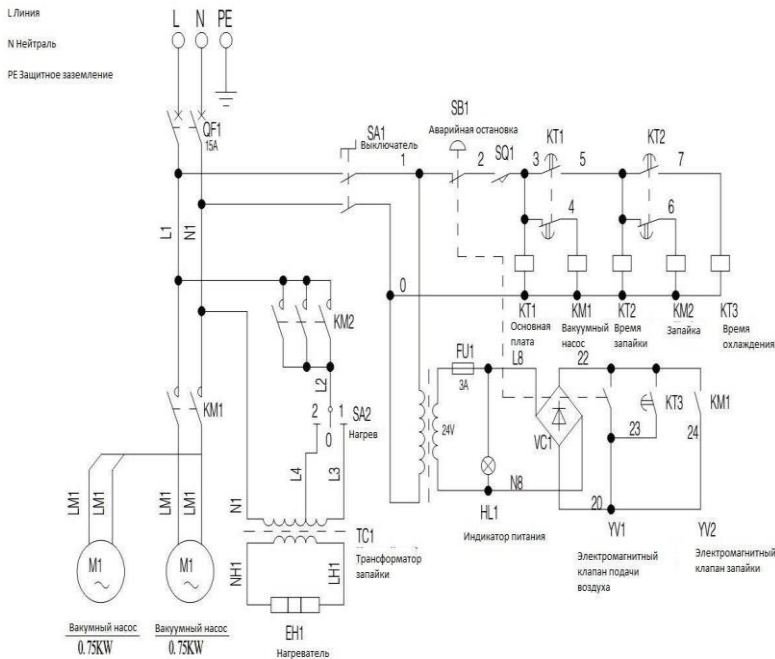
Однофазная схема (220В 50Гц)
